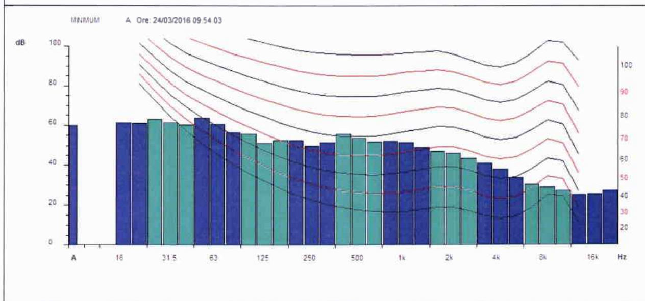
Profilo temporale L_{AFmax} e spettro in frequenza in terzi di ottava relativi alla misura nel punto A_1
